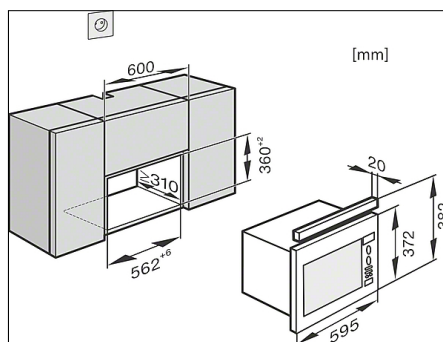
M6030SC, M6032SC, överskåp, 60 cm bred med AB36 (skiss)
