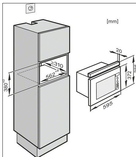
M6030SC, M6032SC, högskåp, 60 cm bred med AB38 (skiss)
