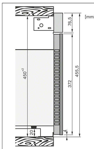
M6030SC, M6032SC, högskåp, 60 cm bred med AB45-9, sidovy (skiss)
