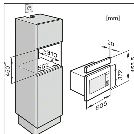
M6030SC, M6032SC, högskåp, 60 cm bred med AB45-9 (skiss)
