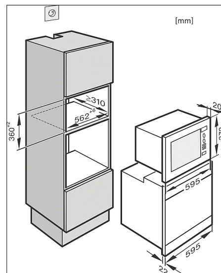
M6030SC, M6032SC, högskåp, 60 cm bred med ugn (skiss)
