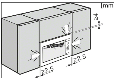
M6022SC, M6030SC, M6032SC, M6040SC, till- och frånluft (skiss)
