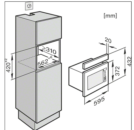
M6030SC, M6032SC, högskåp, 60 cm bred med AB42 (skiss)
