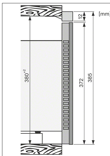
M6030SC, M6032SC, högskåp, 60 cm bred med AB38, sidovy (skiss)
