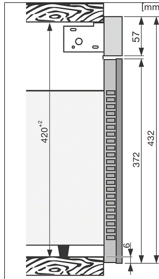
M6030SC, M6032SC, högskåp, 60 cm bred med AB42, sidovy (skiss)
