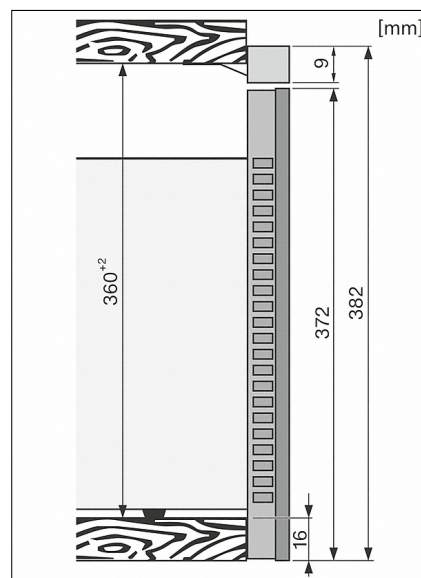
M6030SC, M6032SC, överskåp, 60 cm bred med AB36 (skiss)
