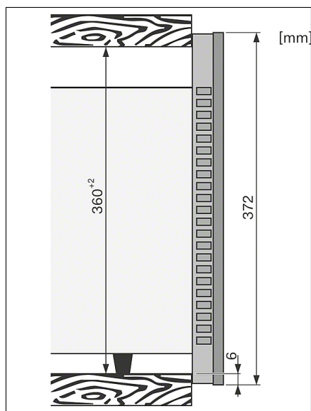
M6030SC, M6032SC, högskåp, 60 cm bred, sidovy (skiss)
