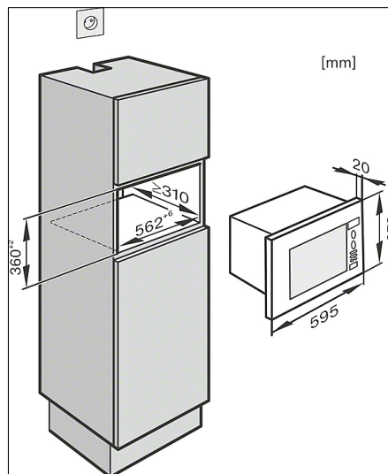
M6030SC, M6032SC, högskåp, 60 cm bred (skiss)
