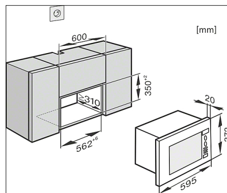
M6030SC, M6032SC, överskåp, 60 cm bred (skiss)
