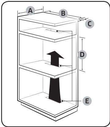
Kaapisto (mm)
