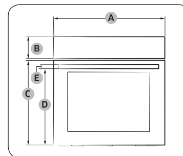
Ovn (mm)
