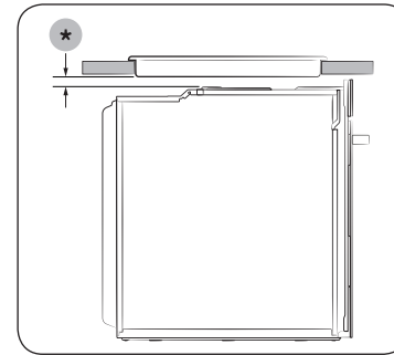
Uunin asentaminen
