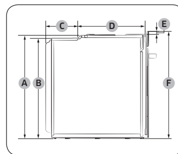
Ugn (mm)
