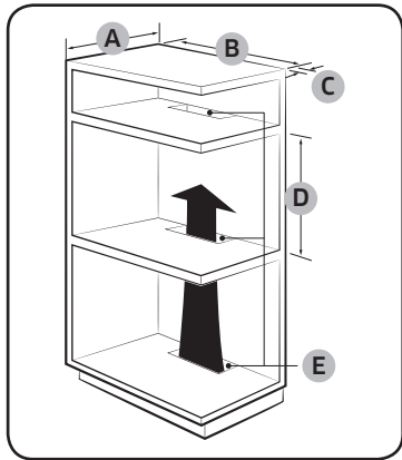
Indbygningsskab (mm)
