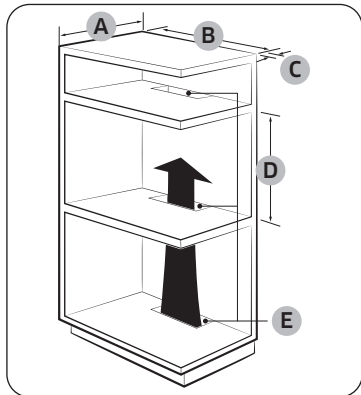
Sisäänrakennettu kaappi (mm)
