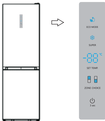
Näyttöpaneeli ovenssa
