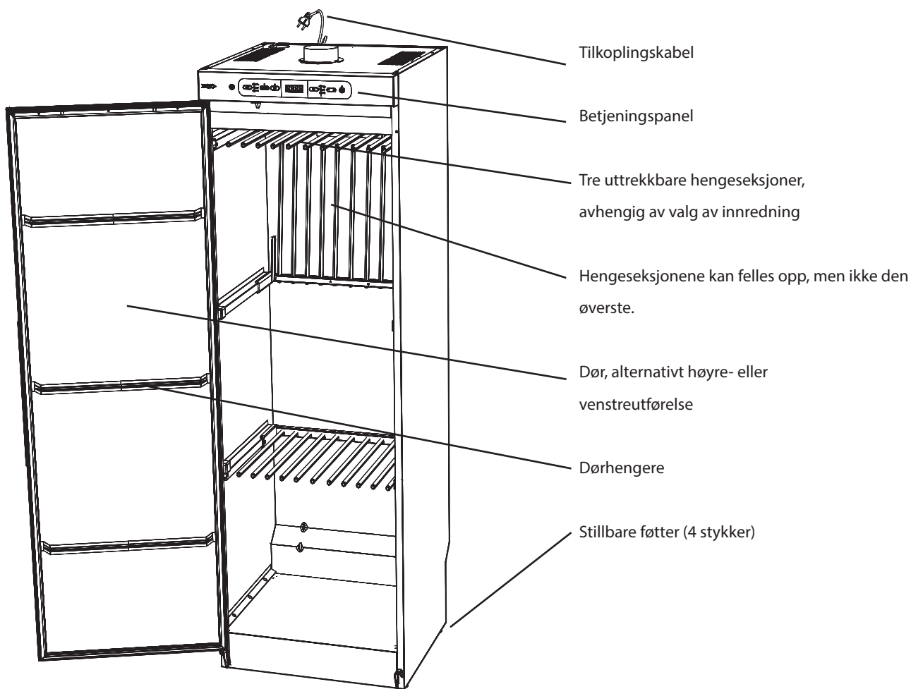
Figuren viser tørkeskap Sensor Dryer
