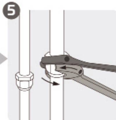
Anslut rörledningar
