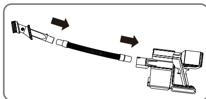
Kuva 10 (nelikulmainen harja/ sähköstaattinen harja) Mahdollisia jatkoputken liitöntäapoja
